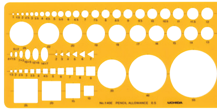
012-0014 No.140E 建築士・受験者用定規 / 1,340円(税込1,474円) ●233×114mm ●厚さ0.8mm ●ブチレート製 ○包装入数1/30 これ1枚で平面図が描ける 課題で要求の多い、10m・8m・6m・5mの内接円を1枚に配置。 柱サイズ：700角800角900角にも対応しています。 (全てS=1/200の場合) 直径40・50mmの大きな円も描けます。
