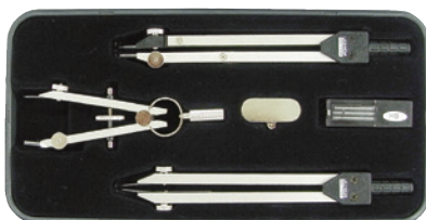
010-0012 KJ7品組 / 6,700円(税込7,370円) ●コンパス(適正使用半径15~110mm) ●デバイダー ●スプリングコンパス小型(鉛筆) ●芯入(2mm芯) ●分度器9cm ●字消板 ●ドライバー ○包装入数1/5/40
