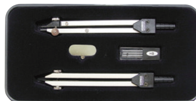
010-0011 KJ6品組 / 4,900円(税込5,390円) ●コンパス ●デバイダー ●芯入(2mm芯) ●分度器9cm ●字消板 ●ドライバー ○包装入数1/5/40
