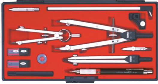
1-730-7413 QB13品組
