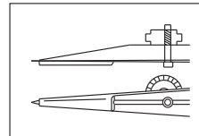
英型大文回(引針式)
